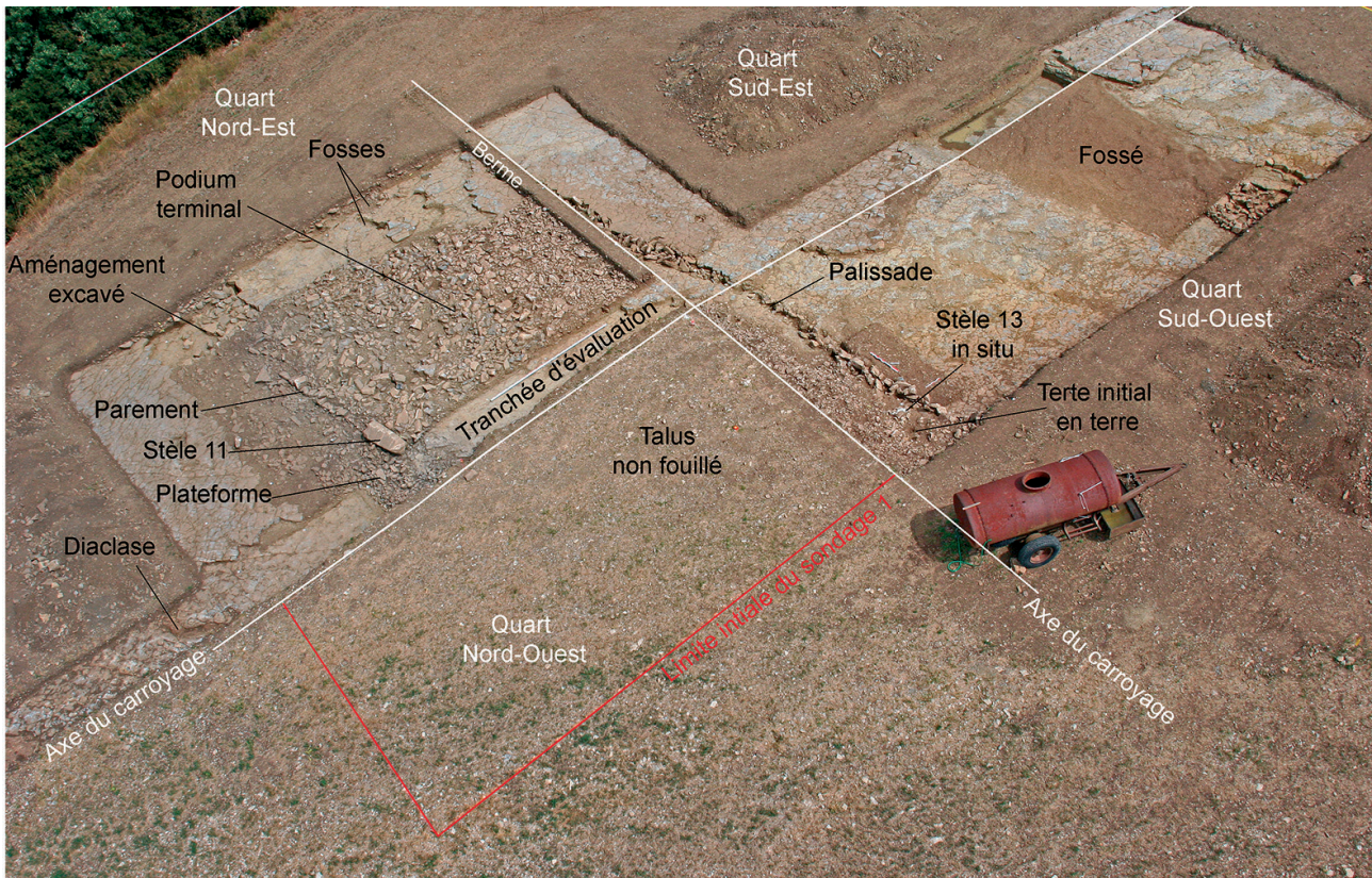
Fig. 2 : Vue oblique du site des Tourières lors de la fouille de 2008 avec la localisation des principales structures mises au jour et les divers secteurs (cliché atelier photo Costes).
